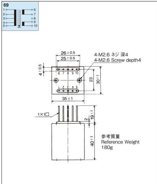
TFP-W Type ケース/結線図 Case / SCHEMATIC
