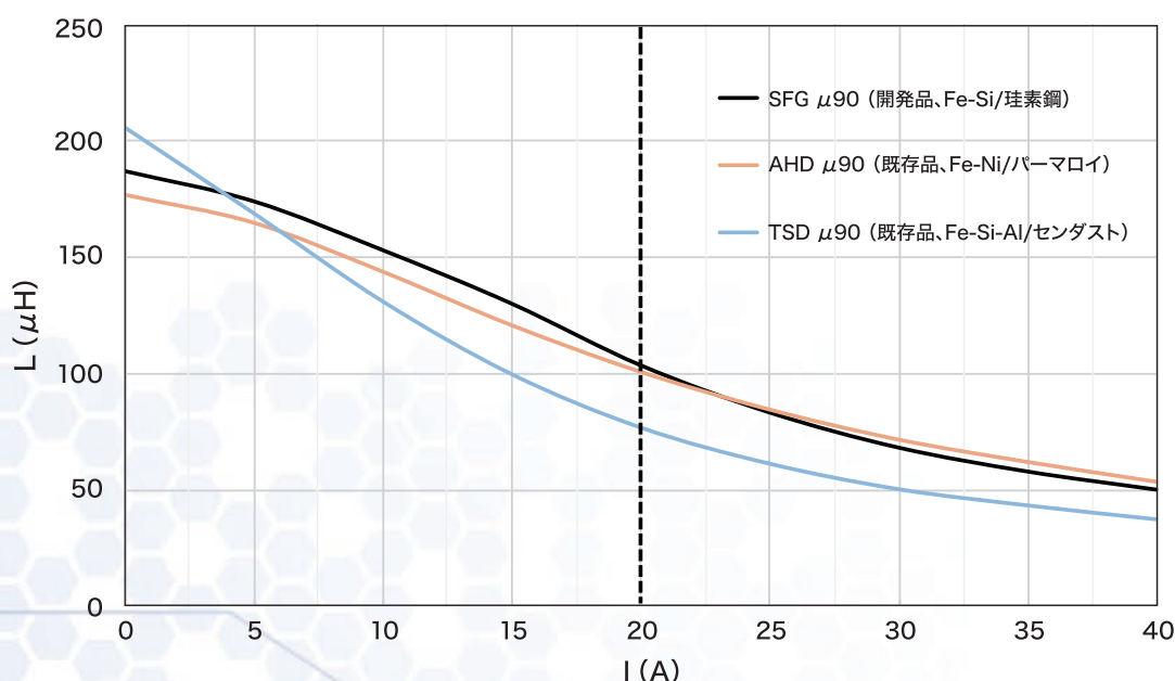
L-I 特性 (定格 20A / Rated 20A)
